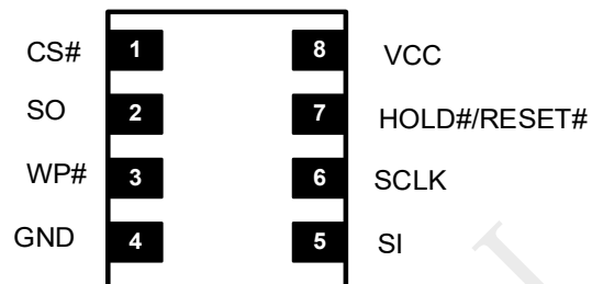
8-Pad USON (1.5x1.5/3x2mm)
